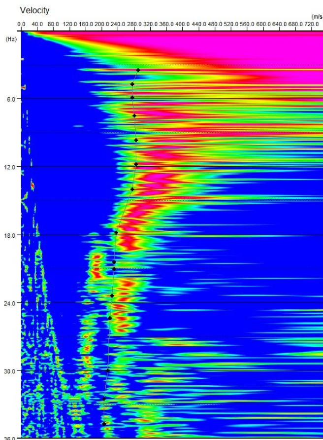
Fig. 15 CURVA DI DISPERSIONE CUMULATIVA METODI ATTIVO E PASSIVO
