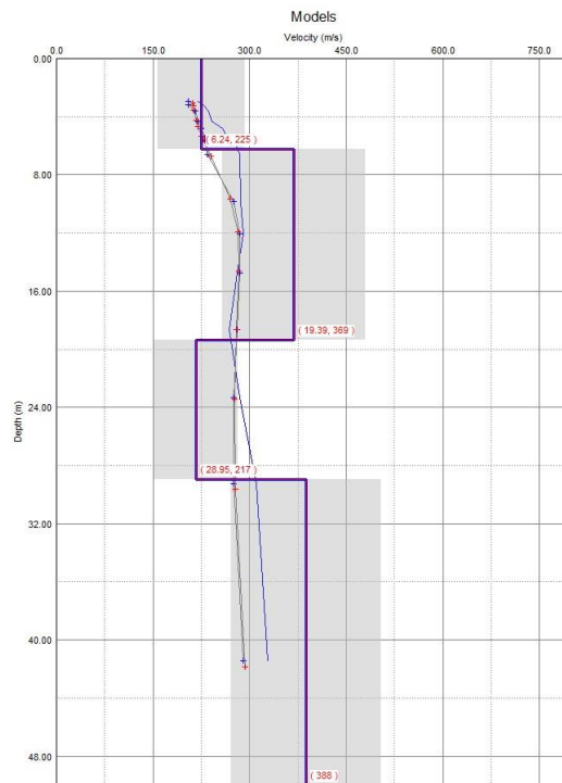
Fig. 17 MODELLO RISULTANTE DALL'INVERSIONE DEI DATI
