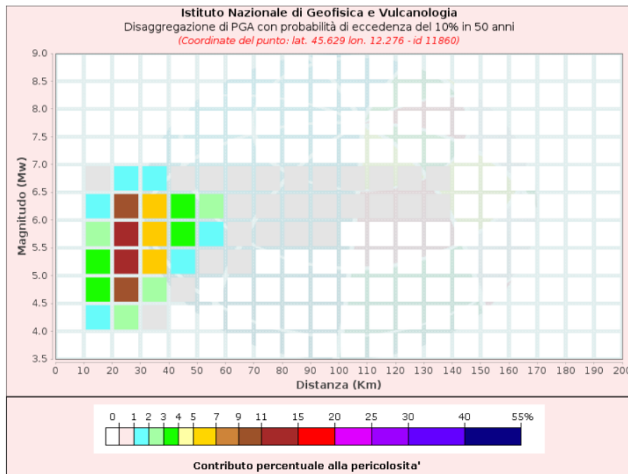
Fig. 23: analisi di disaggregazione del sito in esame (SLV)
