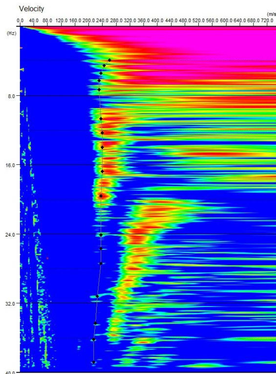
Fig. 18 CURVA DI DISPERSIONE CUMULATIVA METODI ATTIVO E PASSIVO
