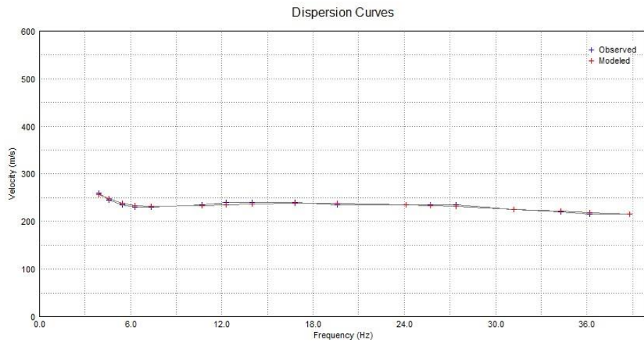
Fig.19 CURVA DI DISPERSIONE MISURATA (BLU) E CALCOLATA (ROSSO)
