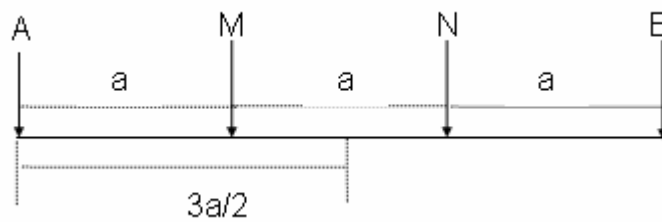
Figura 13 Schematizzazione del dispositivo quadripolare tipo WENNER, comunemente utilizzato per l'acquisizione di dati di resistività elettrica. AB: elettrodi di corrente; MN: elettrodi di potenziale.
