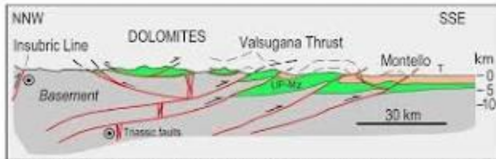
Fig.5 Sezione del ventaglio embriciato delle Alpi Meridionali, dalla Val Pusteria alla pianura veneta (da Doglioni & Carminati, 2008). La zona in studio si trova a Sud del rilievo del "Montello".
